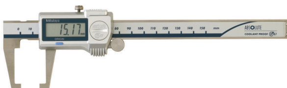
573-651-20 avec becs intérieurs pour mesurer l'épaisseur des parois
