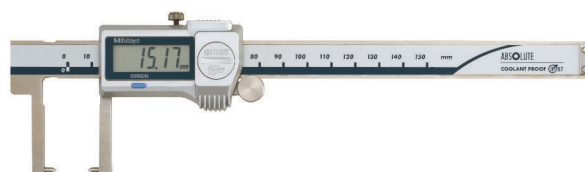
573-652-20 avec pointes de mesure intérieure
